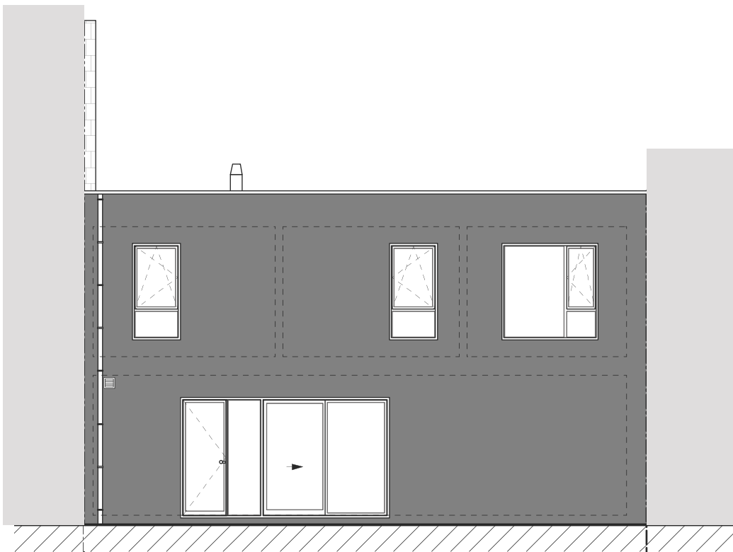
ACHTERGEVEL
