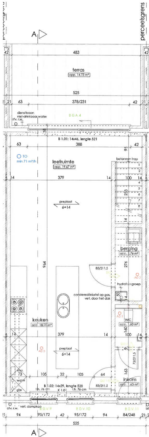
plan gelijkvloers woning B4 huisnr. 56 opp. gelijkvloers excl. tuinmuur : 54.60 m²
