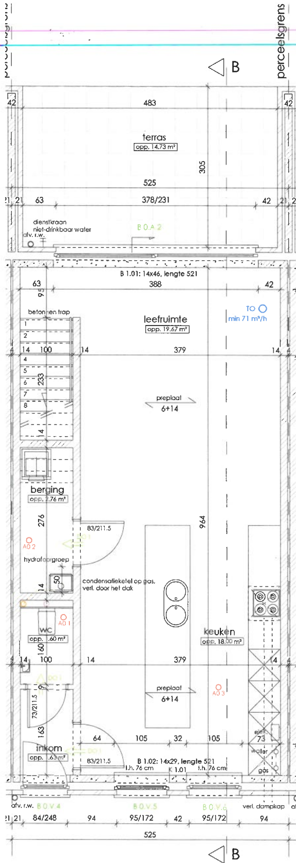
plan gelijkvloers woning B2 huisnr. 52 opp. gelijkvloers excl. tuinmuur : 54.60 m²
