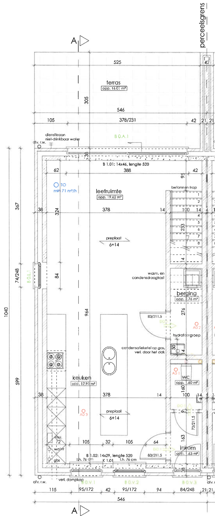
plan gelijkvloers woning B1 huisnr. 50 opp. gelijkvloers excl. tuinmuur : 56.78 m²
