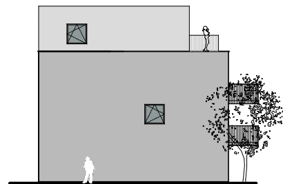
ZIJGEVEL west
